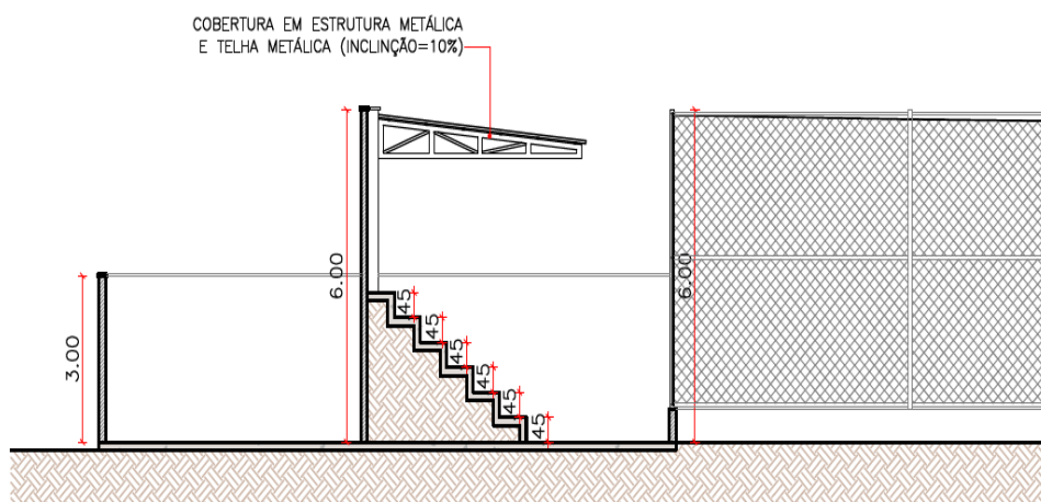
CORTE AA'
